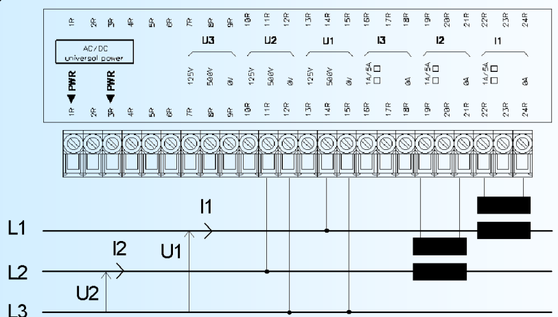
TRIPHASE DESEQUILIBRE SANS NEUTRE Méthode des deux wattmetres avec I1 et I2 disponibles
