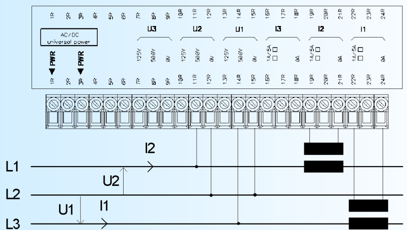
TRIPHASE DESEQUILIBRE SANS NEUTRE Méthode des deux wattmetres avec I1 et I3 disponibles
