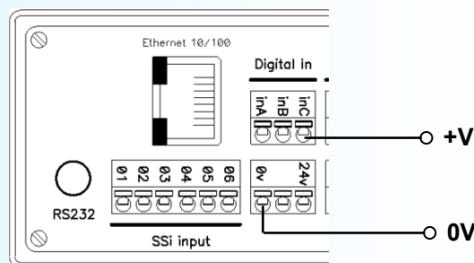
Entrée tension
