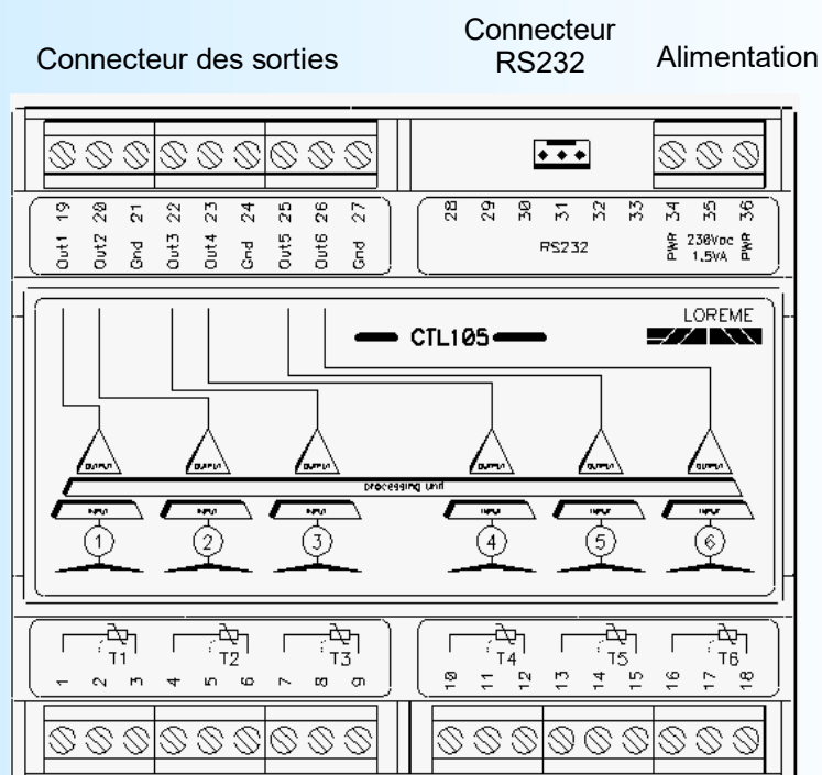
Connecteurs des entrées 1 à 6.
