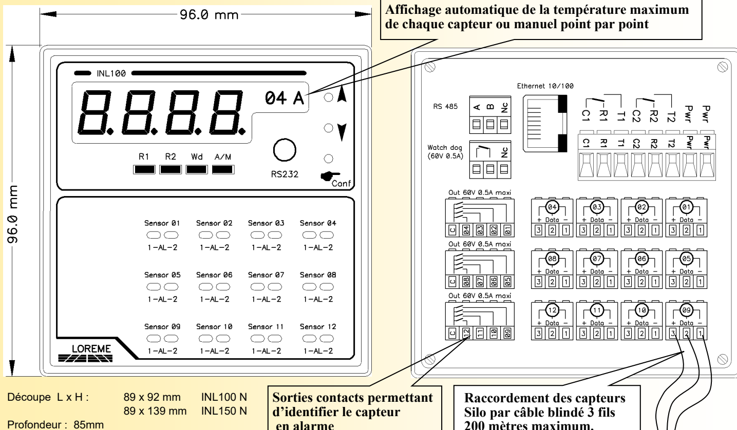
Capteur Silo numérique Type Siloflex-N 24 points de température maximum
