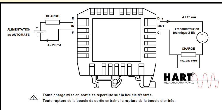
Utilisation du CAL25IGA pour l'isolation d'un transmetteur en technique 2 fils
