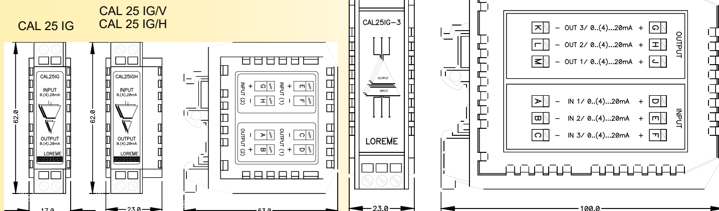
Utilisation de CAL25IG, IG3, IG/V pour l'isolation d'une charge
