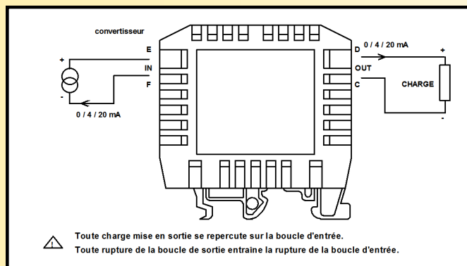
Utilisation de CAL25IG, IG3, IG/V pour l'isolation d'une charge
