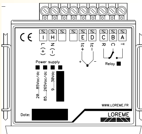
Version entrée Thermocouple
