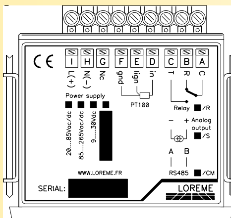
Version entrée PT100, PT1000
