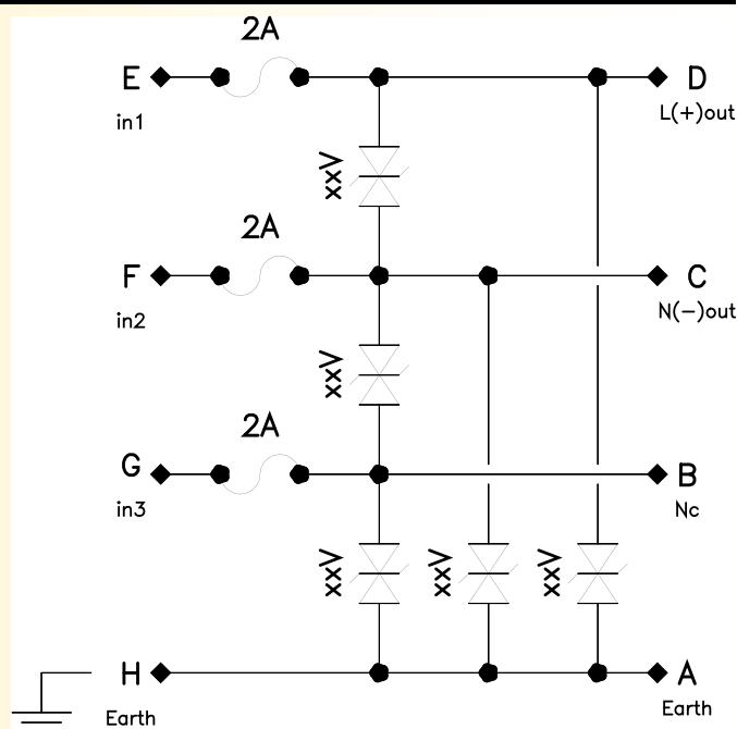
Schéma interne version PFL25-TVS (PARASURTENSEUR)
