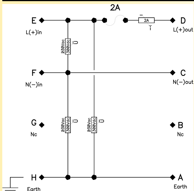
Schéma interne version PFL25-MOV (PARAFOUDRE)
